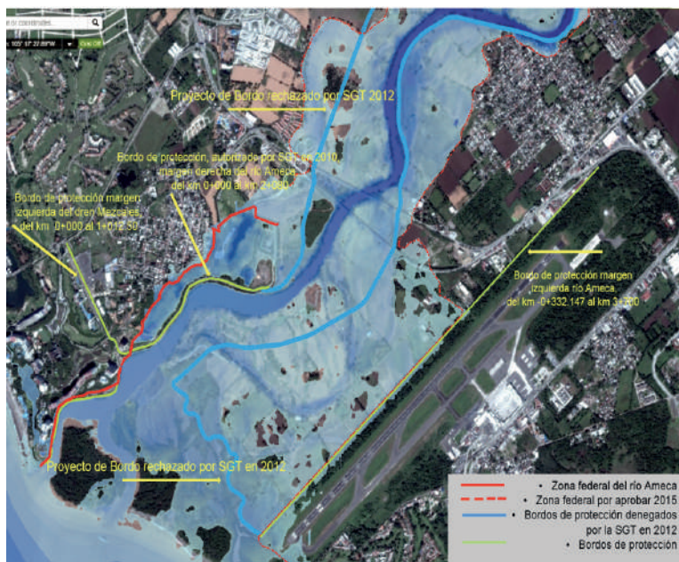
FIGURA 10.5. MODELACIÓN BIDIMENSIONAL DEL RÍO AMECA ANTE LA OCURRENCIA DEL HURACÁN PATRICIA EN 2015. (FUENTE: SGT)
