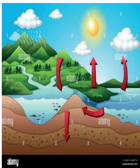
FIGURA 6.1. CICLO HIDROLÓGICO (CORTESÍA DE ALAMY)
