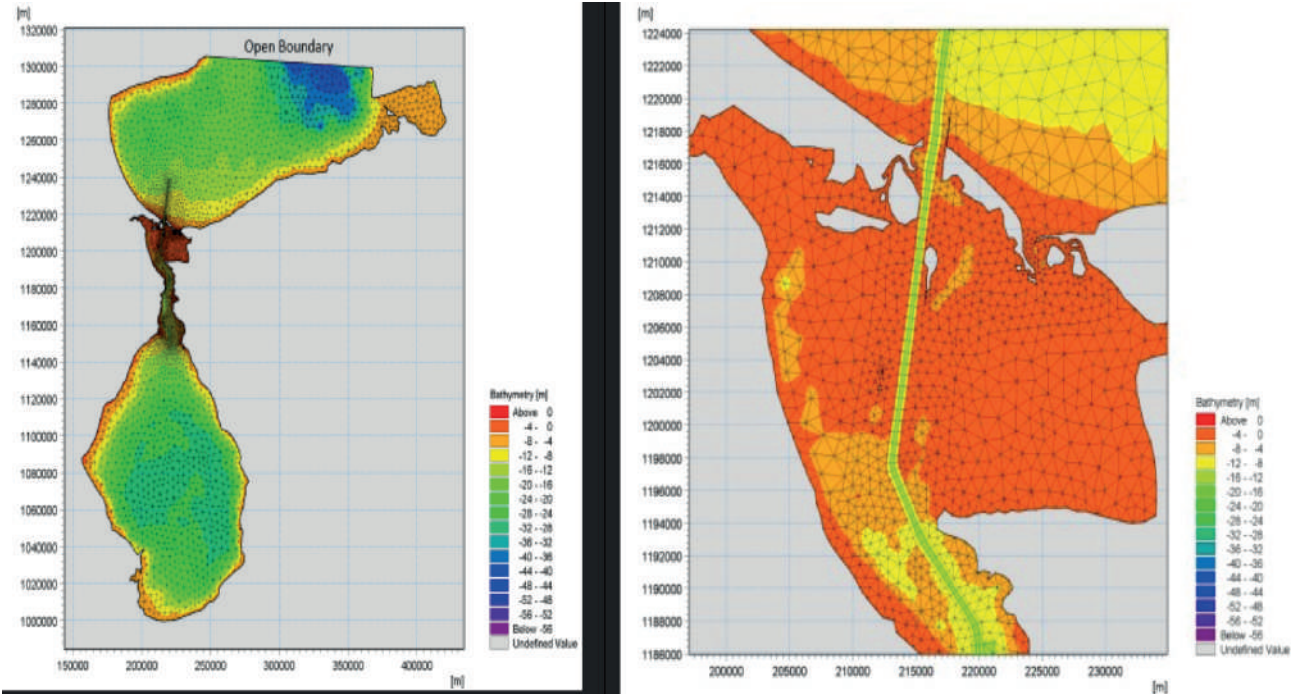
FIGURA 8.10. BATIMETRÍA LAGO MARACAIBO
