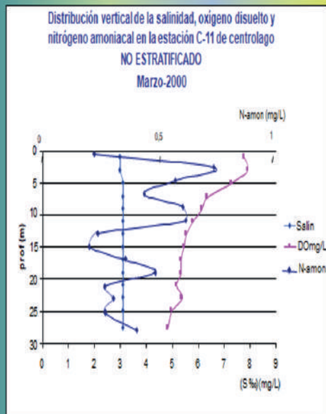
FIGURA 8.11. DISTRIBUCIÓN VERTICAL NO ESTRATIFICADA DE LA SALINIDAD, OXÍGENO DISUELTO Y NITRÓGENO AMONICAL
