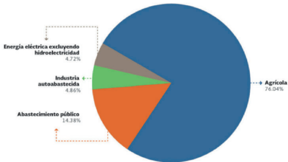
FIGURA 7.2. USOS CONSUNTIVOS DEL AGUA EN MÉXICO.
