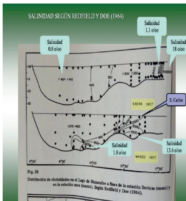
FIGURA 8.7. SALINIDAD LAGO MARACAIBO
