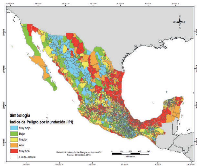
FIGURA 10.2. MAPA DEL ÍNDICE DE PELIGRO POR INUNDACIÓN.
