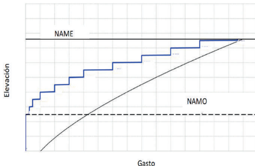
FIGURA 10.4. POLÍTICA DE OPERACIÓN TÍPICA (FUENTE: SGT)
