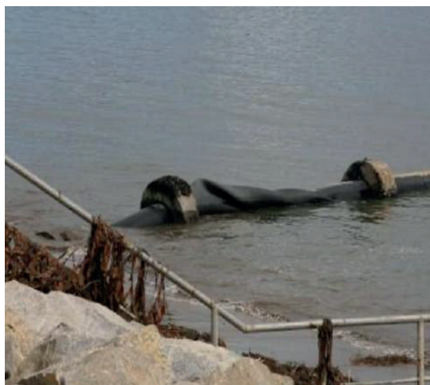
FIGURA 9.4. EMISARIO DE PENCO/LIRQUÉN (600 MM)
