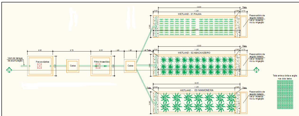
Figura 2: Croqui esquemático da ETE estudada – ETE Aterro – Lagoa D’Anta/RN.
