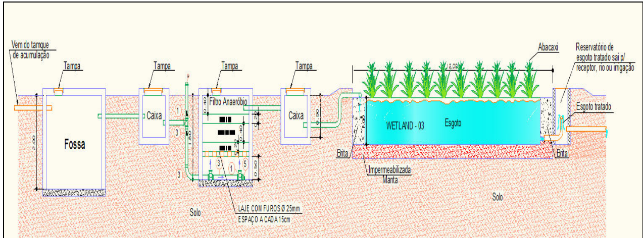
Figura 1: Corte esquemático do sistema estudado.
